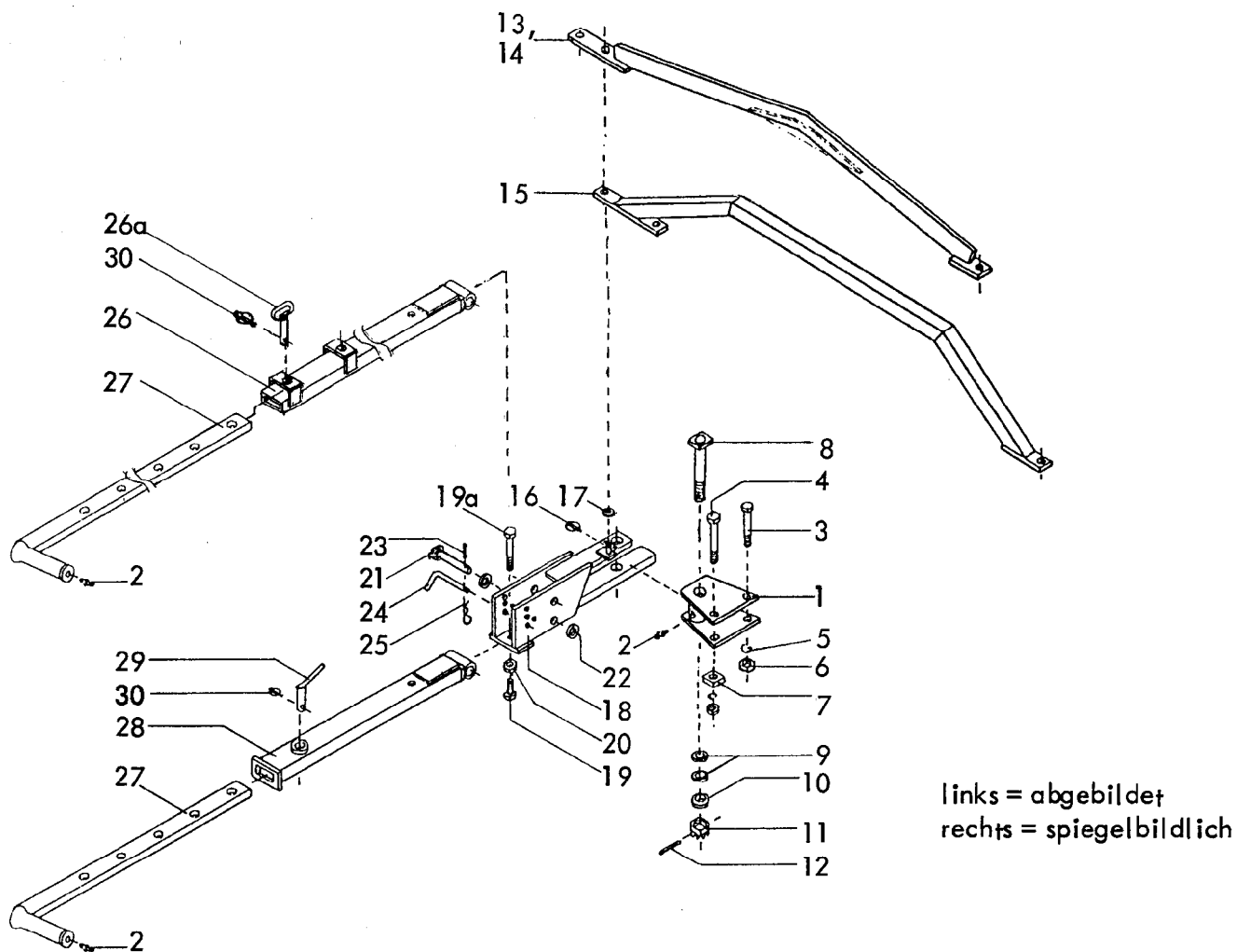
Gerätetyp: Fanghaken für Untergrundpacker, W - Ausführung
