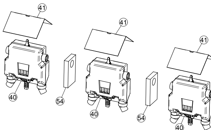
CONFIGURAZIONE C 5 - 6 USCITE SERBATOIO 100-180 dmc
