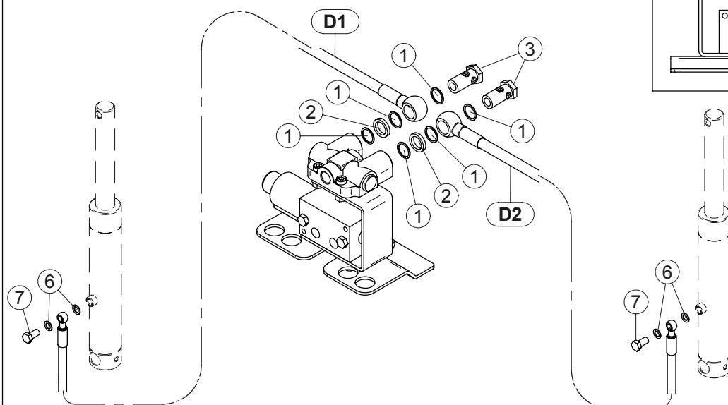
Meccanismo cilindro seminari X230 per telai (250/400-430) - (300/445) - (300/590) - (320/610)
