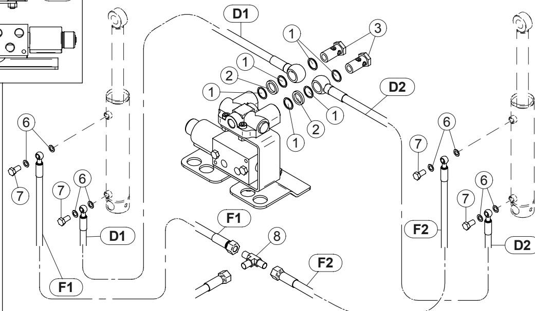
Mecc. cilindri ripieg. bracci X230 per telai (250/400-430) (300/445) (300/590) (320/610)
