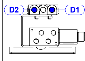
Hydraulisch Anschlusse MS-X230 für Rahmen (250/400-430) - (300/445)
