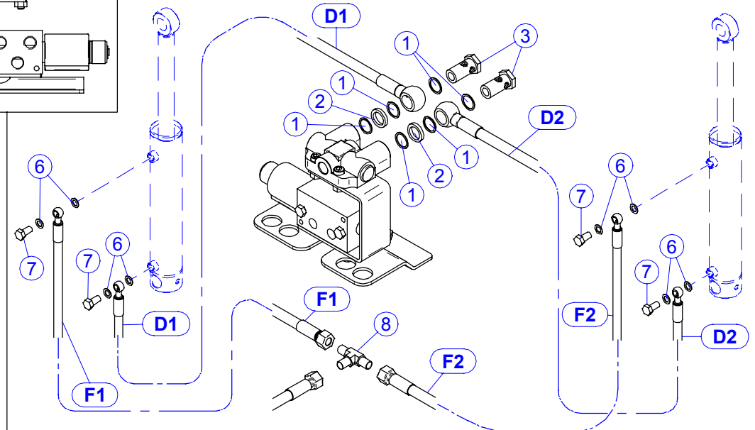
Hydraulisch Anschlusse X230 für Rahmen (250/400-430) (300/445) (300/590) (320/610)
