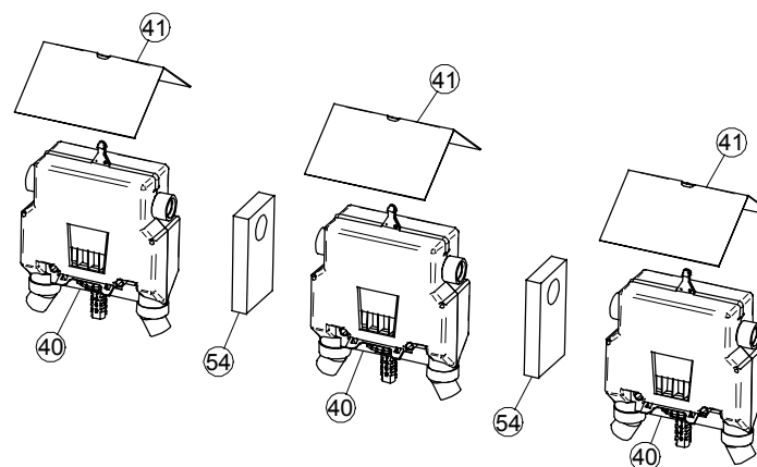
Konfiguration C 5 - 6 Ausläufe Düngerbehälter 100-180 dmc
