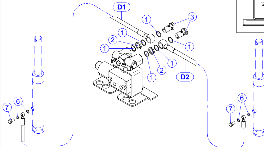
Hydraulisch Anschlusse für Rahmenzylinder MS-X230 (250/400-430) - (300/445) - (300/590) - (320/610)
