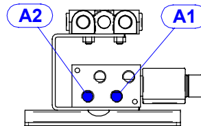
Hydraulisch Anschlusse für Rahmenzylinder MS-X230 (250/400-430) - (300/445) - (300/590) - (320/610)
