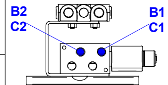
Hydraulisch Anschlusse X230 für Rahmen (250/400-430) (300/445) (300/590) (320/610)
