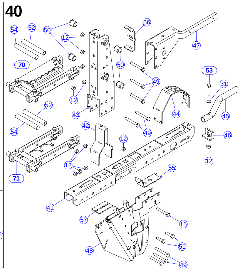
BLOCCO PARALLELOGRAMMA
