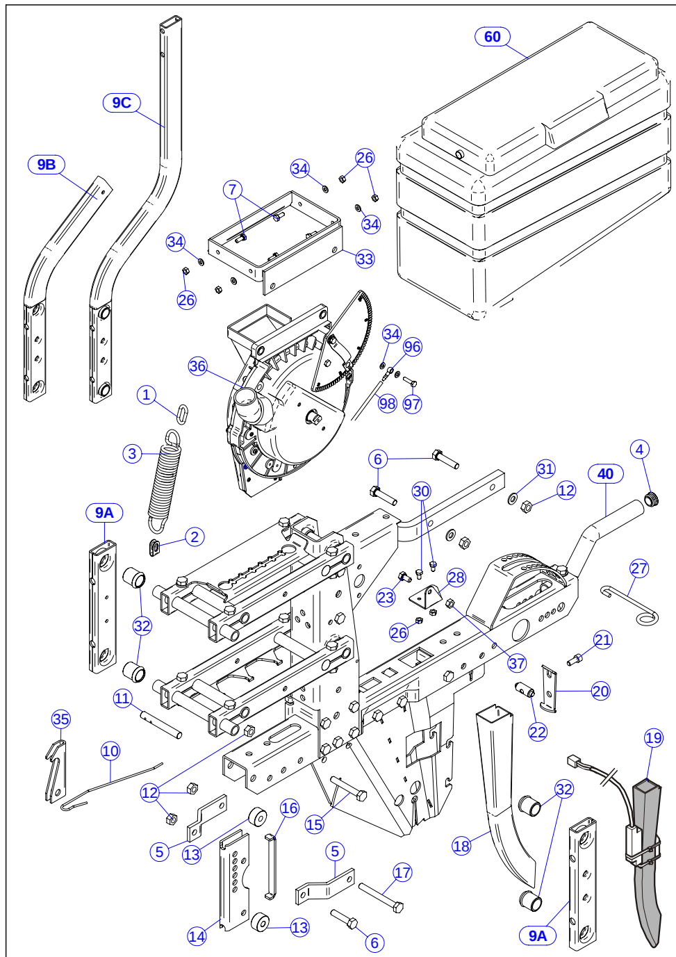
BLOCCO PARALLELOGRAMMA
