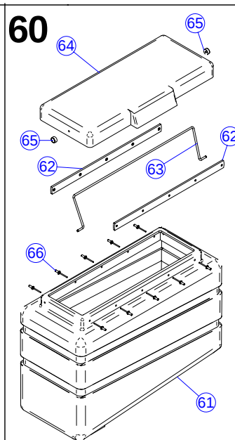
BLOCCO PARALLELOGRAMMA
