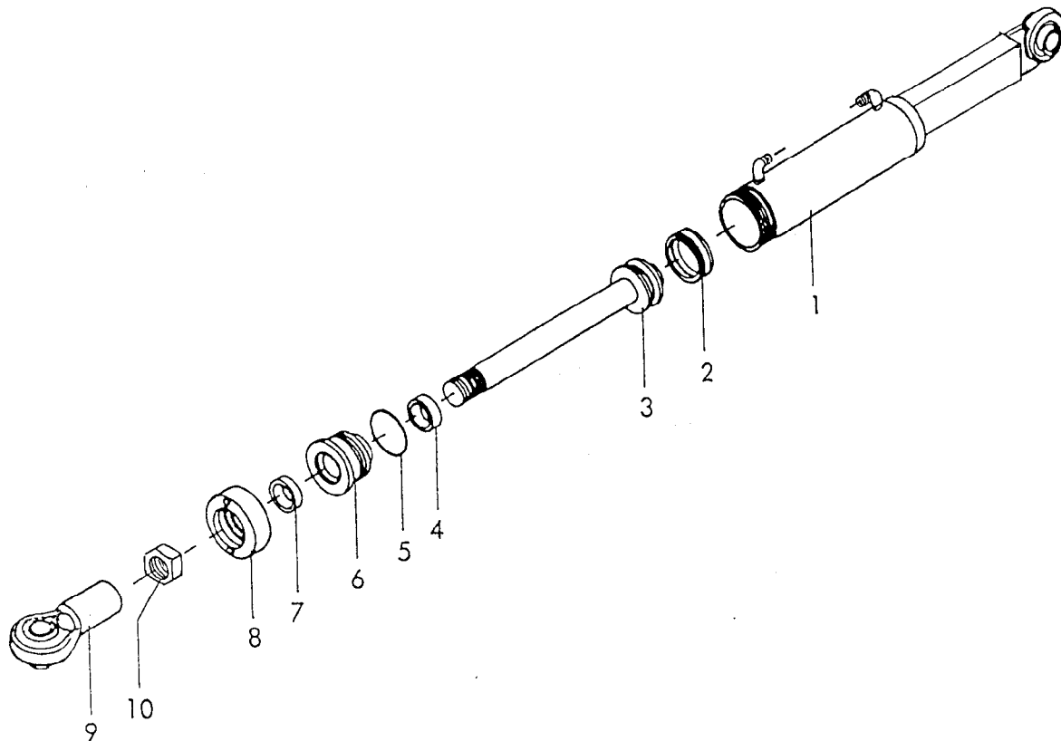
Gerätetyp: Klappzylinder Ø 80 -doppeltwirkend- für XF-600
