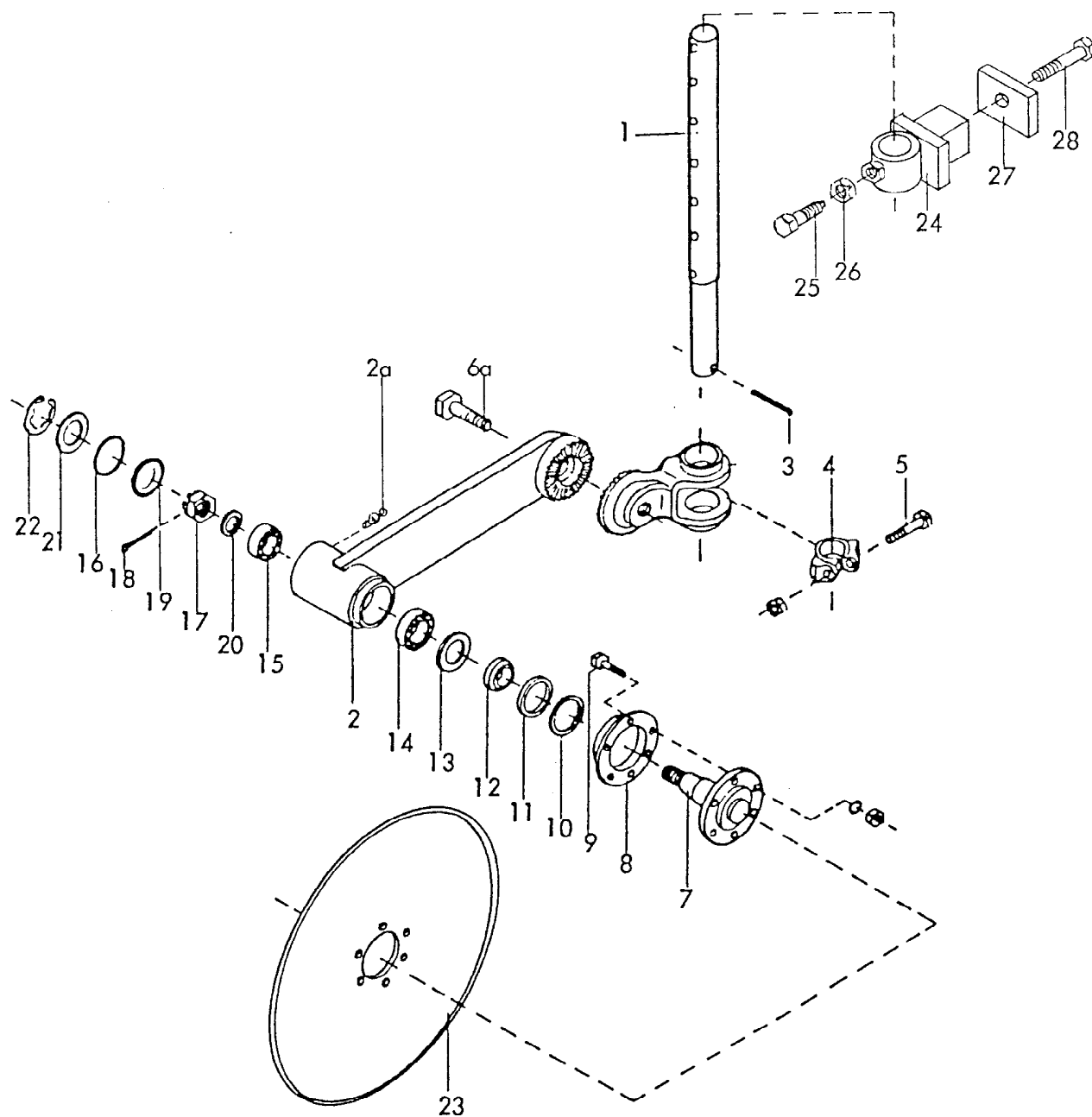
Gerätetyp: Scheibensech " Dok " Ø 400 für Würger I/80
